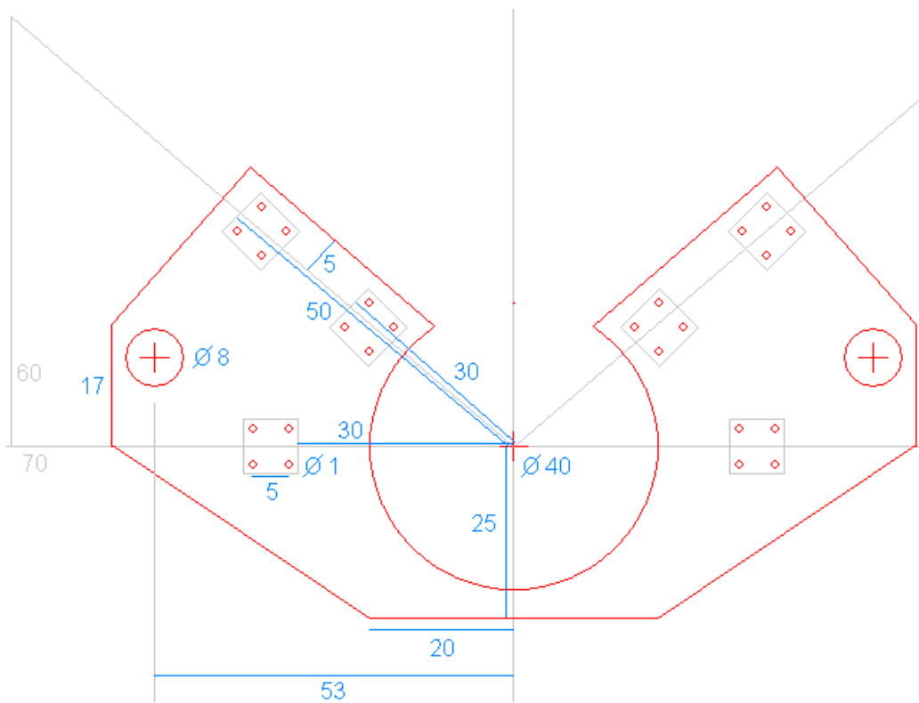
LED-Träger, skaliert (auf DIN A4 ausdrucken)
